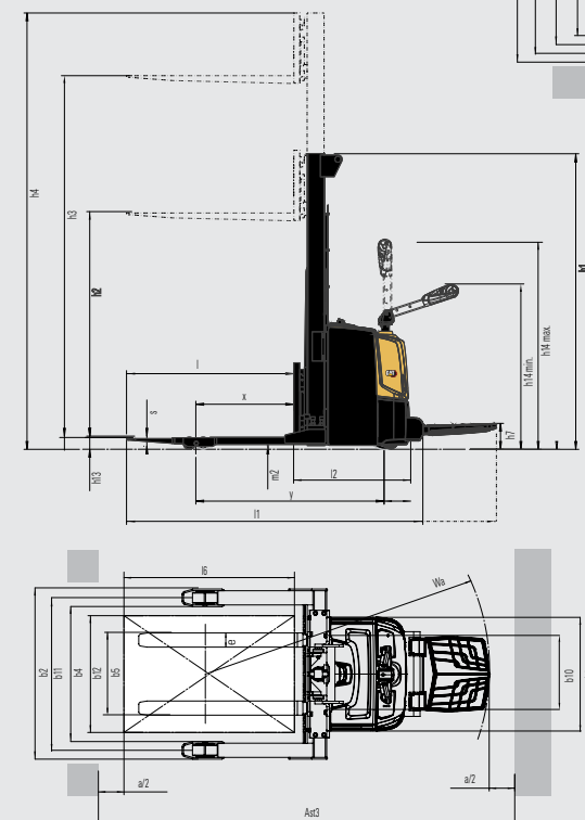
NSP16N2SR: Met opklapbaar platform
