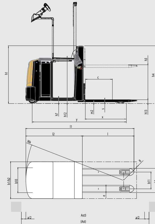
N012N2F: Med höjbara gafflar (N012N2FP: Med höjbara gafflar och plattform)
